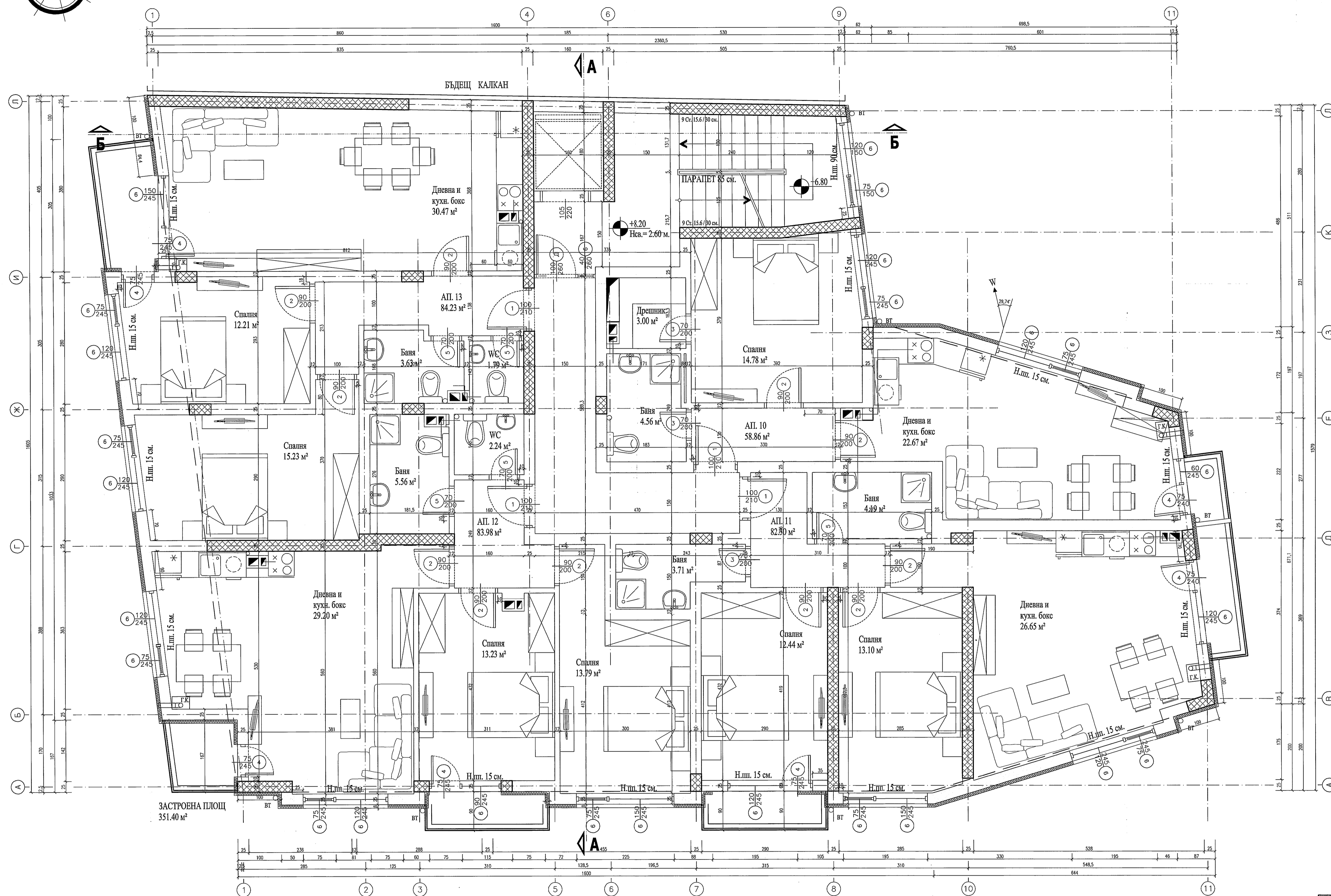
РАЗПРЕДЕЛЕНИЕ КОТА +8.20
